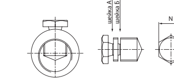
Соединители болтовые рядные с двумя болтами
